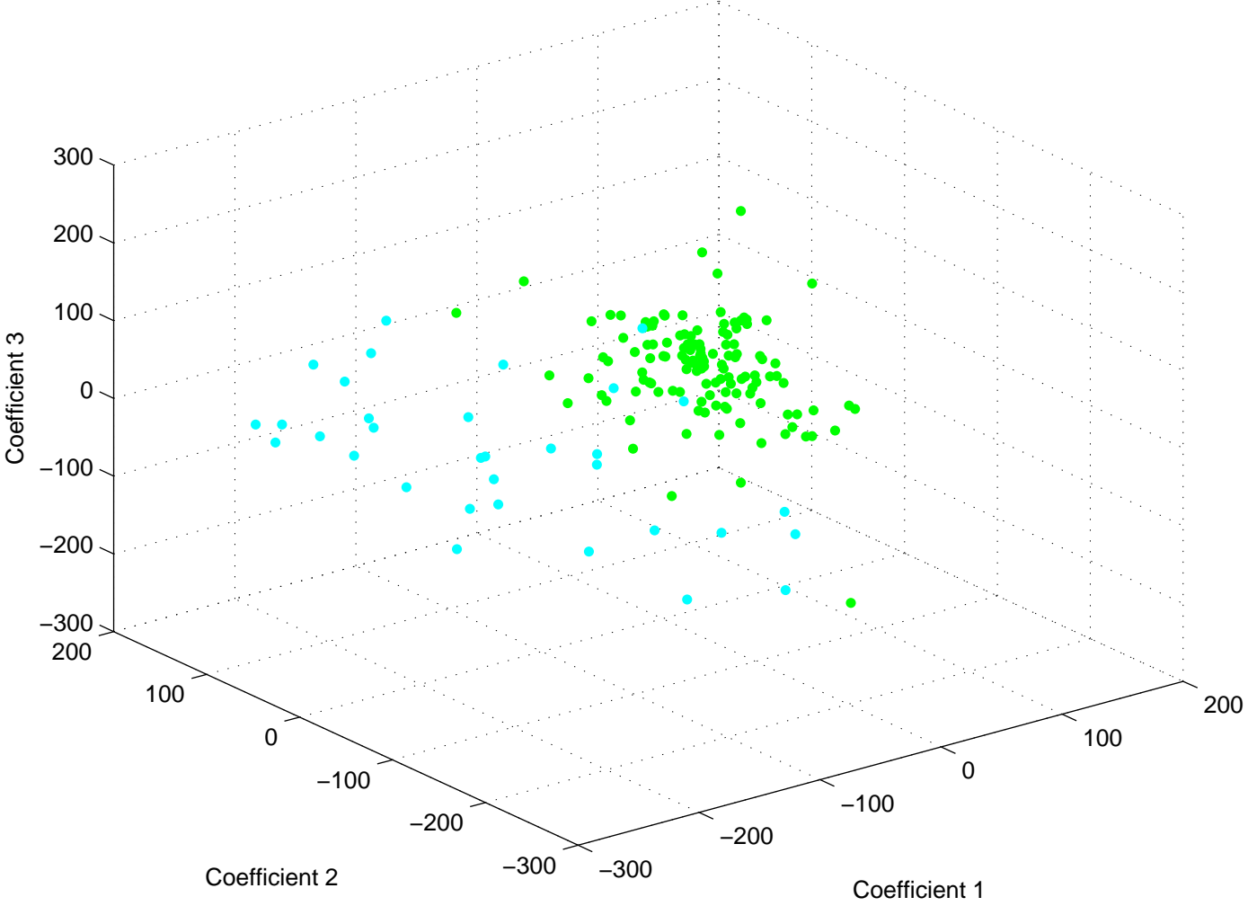
6E6PCA Clustering
